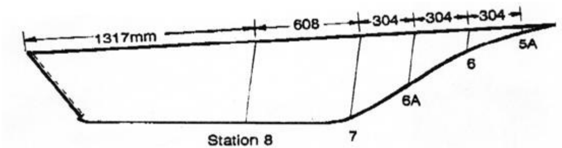
Keel Measurement
